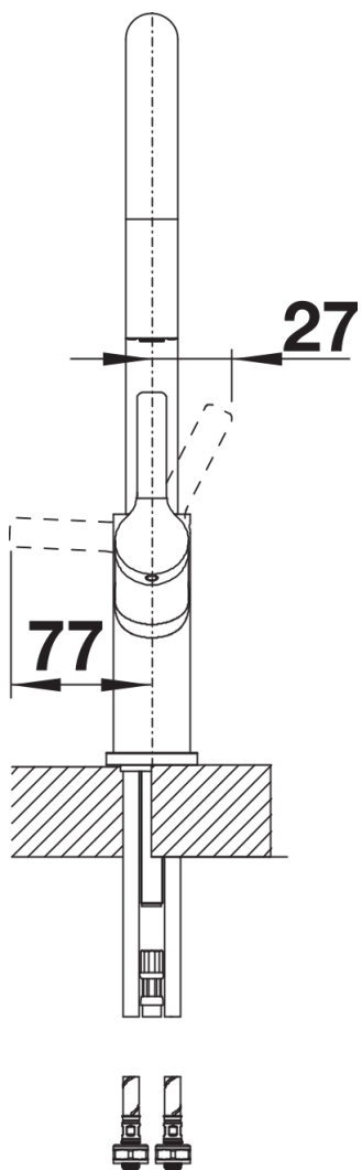
Seitenansicht Hebel 2D
