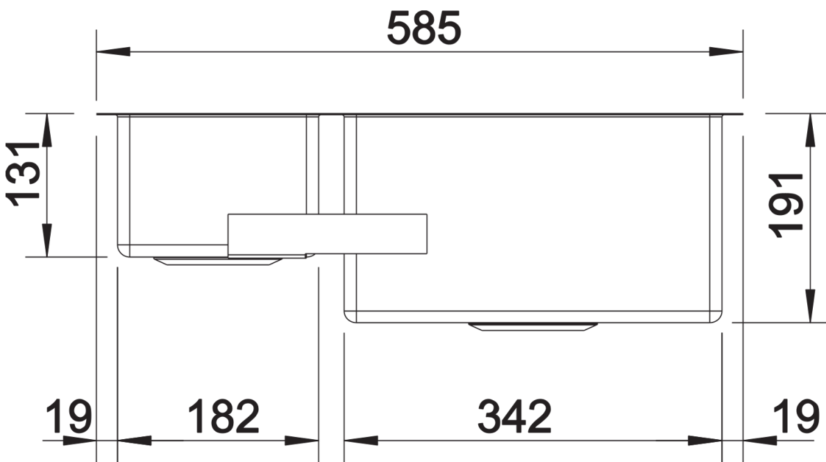
Frontansicht
