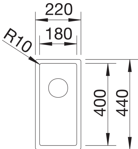
Aufsicht
