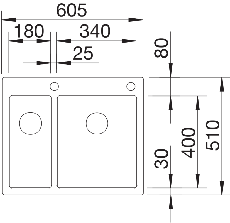
Aufsicht
