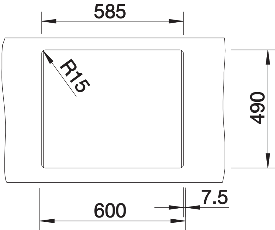
Ausschnitt
