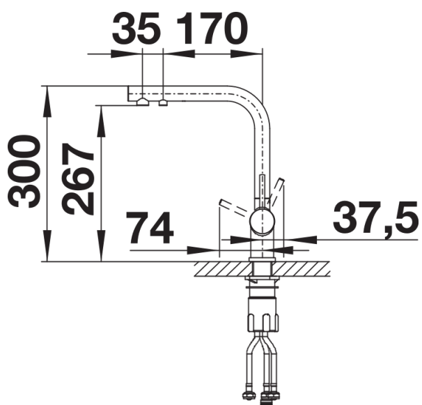
Seitenansicht
