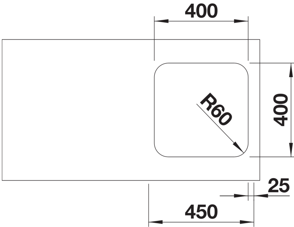
Ausschnitt
