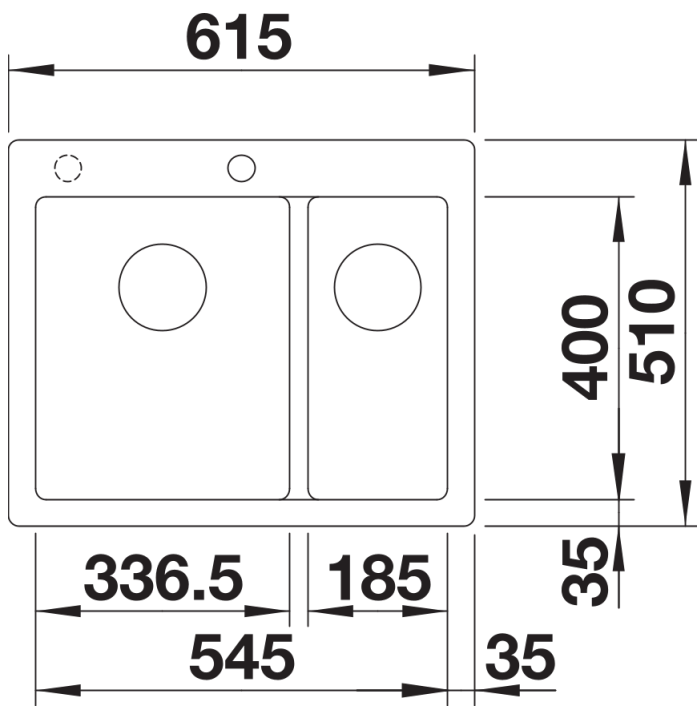
Aufsicht
