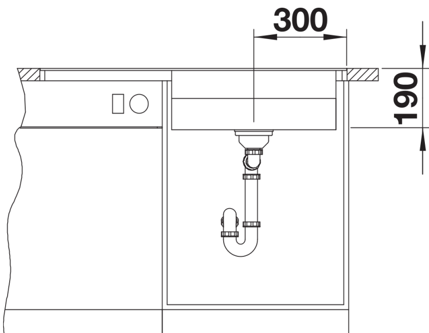
Frontansicht
